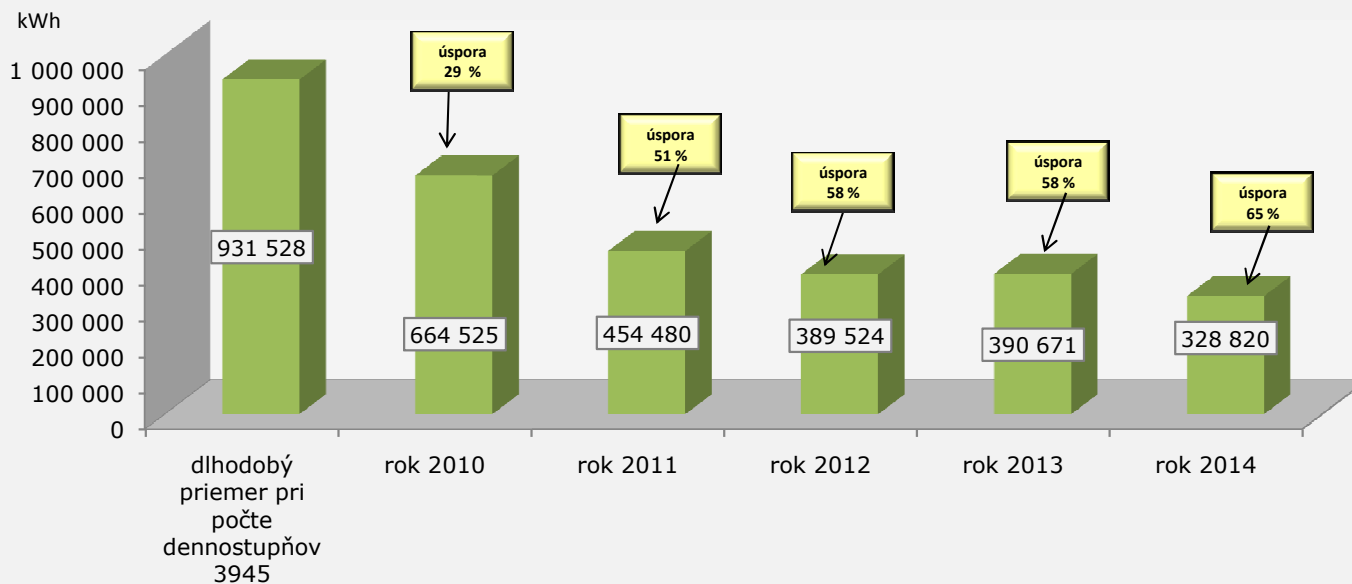
Porovnanie spotrieb tepla na vykurovanie (kWh) - r. 2010-2014
