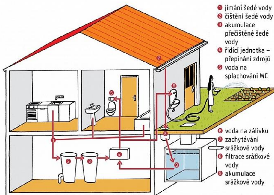
Obrázek 3 - Schéma možného využití šedé vody v kombinaci s HDV
