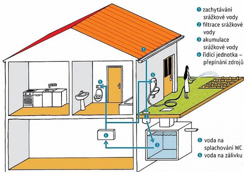
Obrázek 2 - Schéma možného využití dešťové vody v objektu
