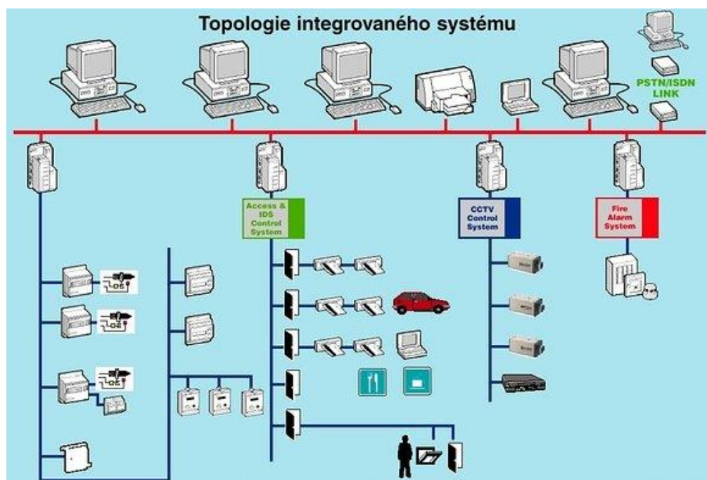
Obrázek 2 - Schéma propojení jednotlivých systémů
